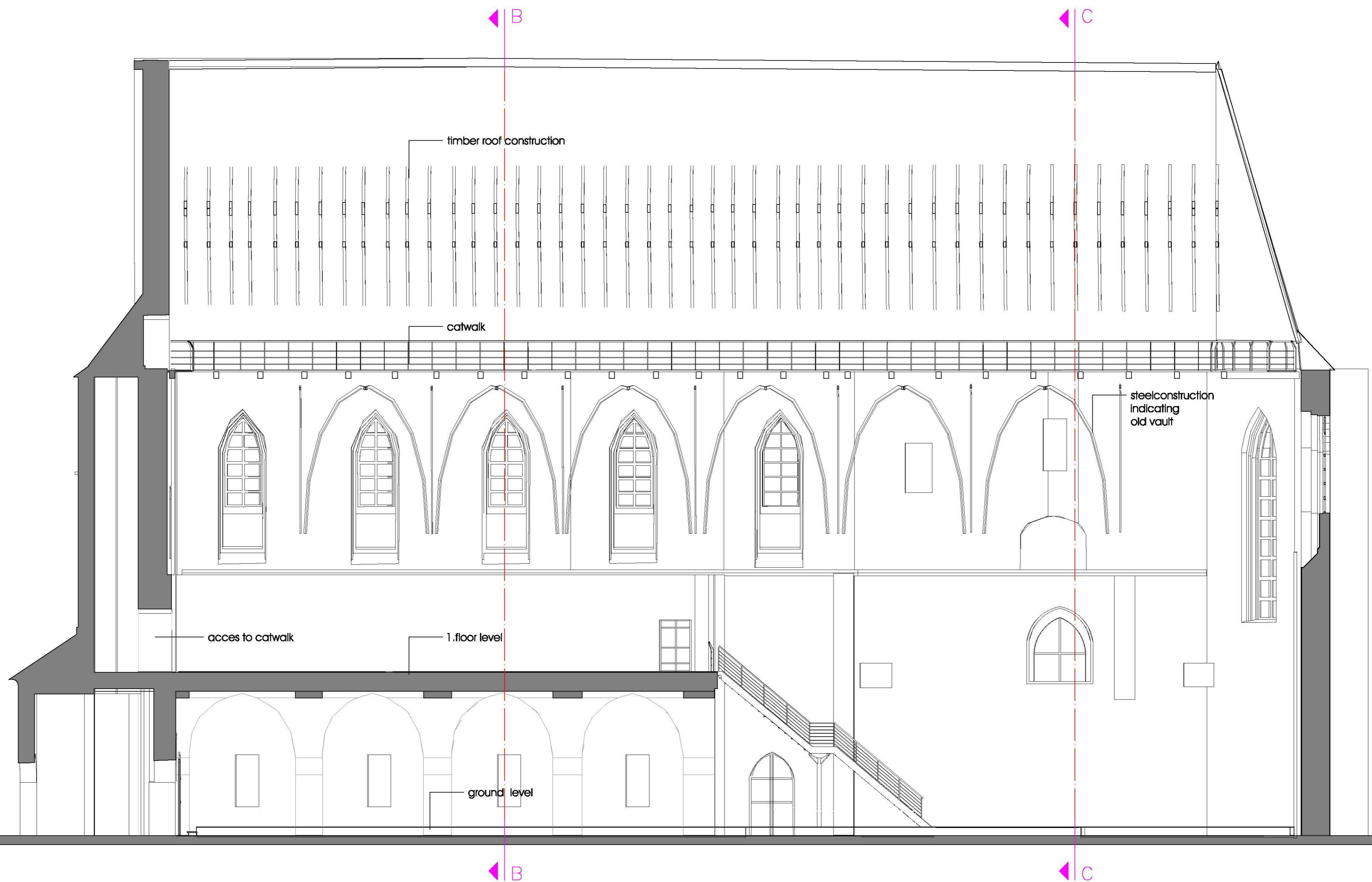
St. Anna Prague longitudinal section A-A
